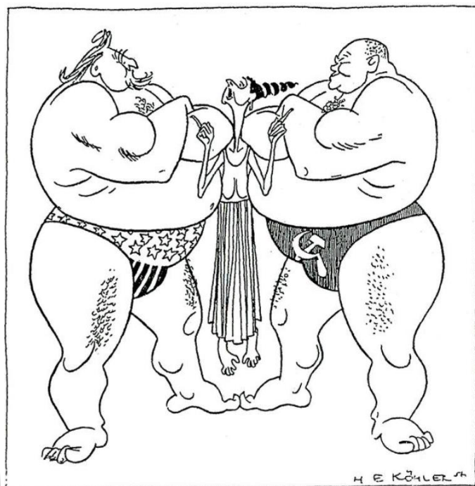
Europa
